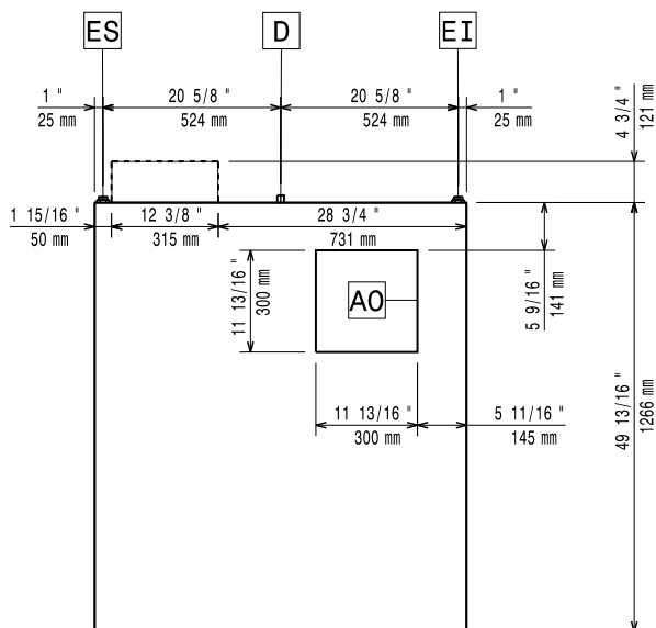
Felülnézet
