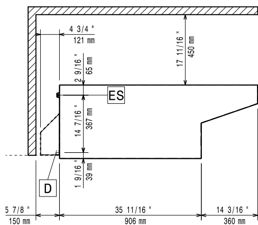
Oldalnézet
